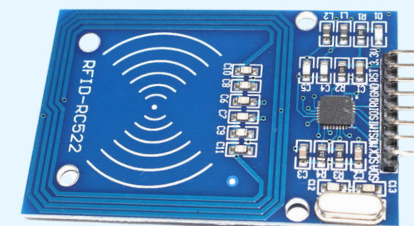
Módulo Leitor Rfid Rc522 Mifare 13,56 Mhz
